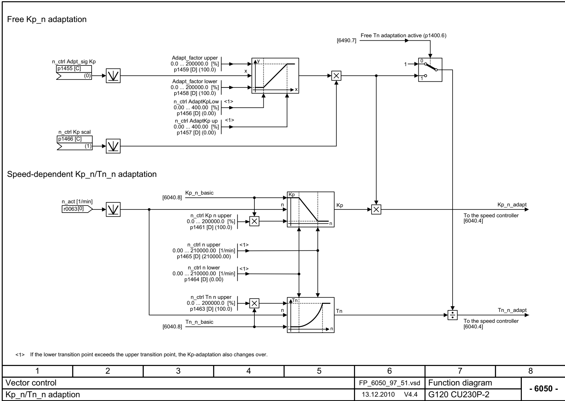
Fig. 2-76 6050 – Kp_n/Tn_n adaption
