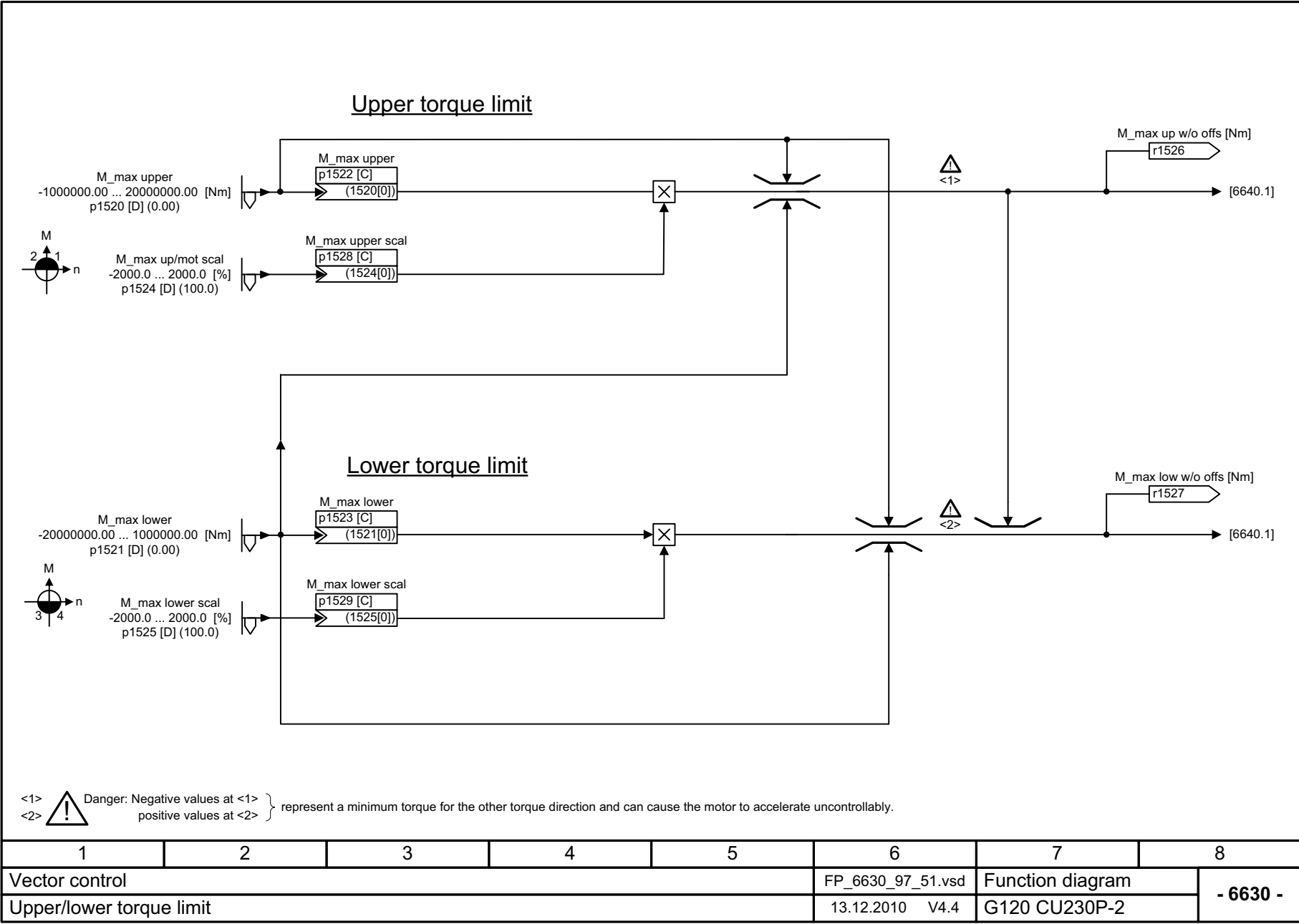
Fig. 2-81 6630 – Upper/lower torque limit
