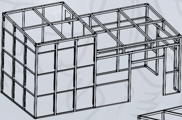
Provedení Kotelny bez Sila
